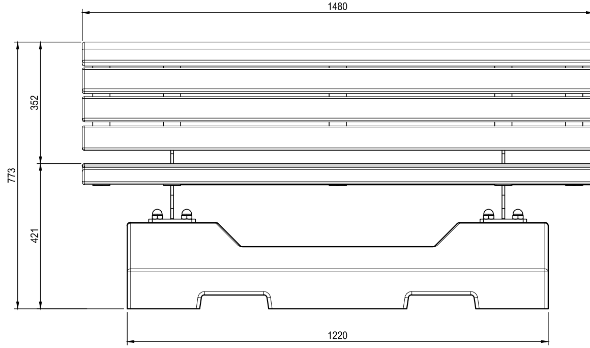
ÖN GÖRÜNÜŞ
